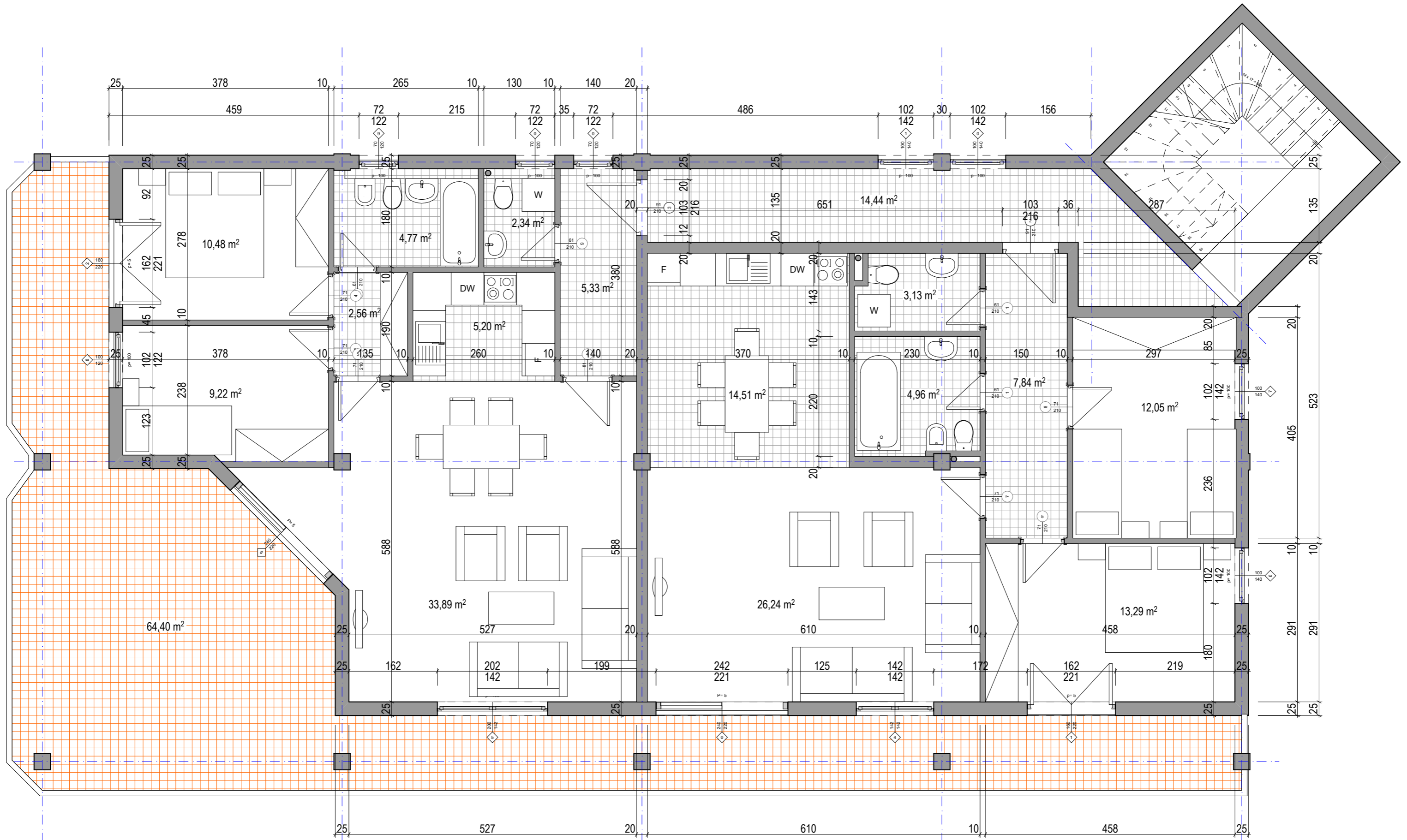
TLOCRT KAT 1 M 1:50
